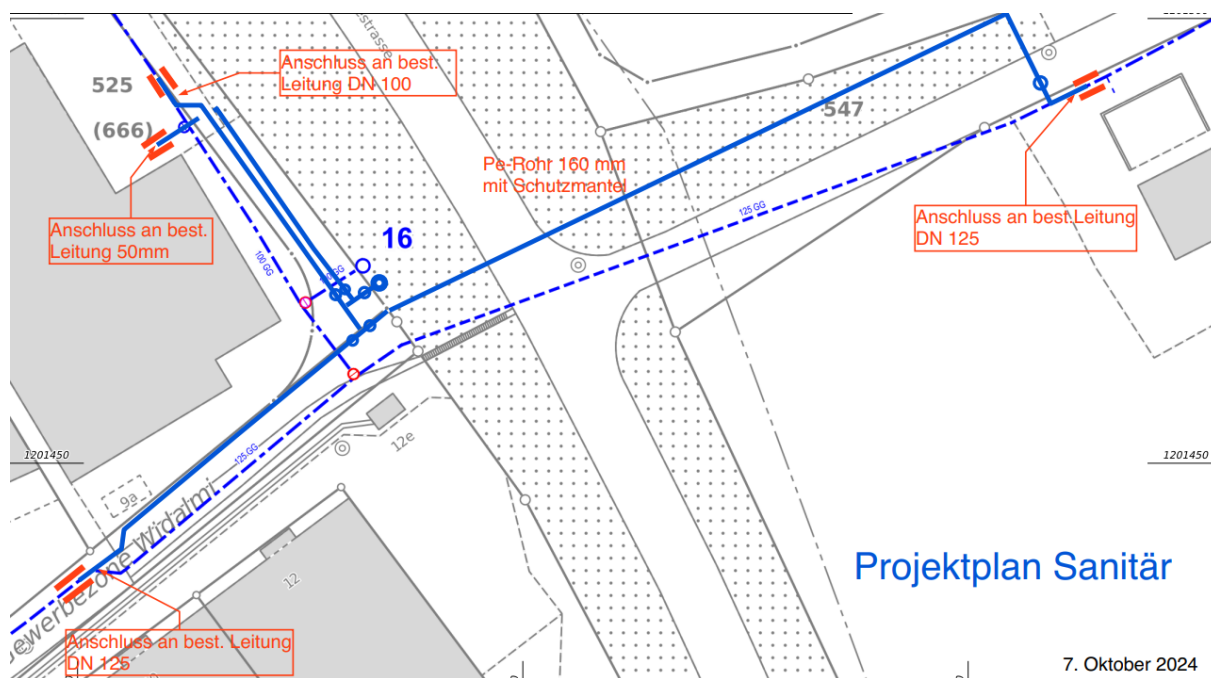
Bild: Projektplan Sanitär
