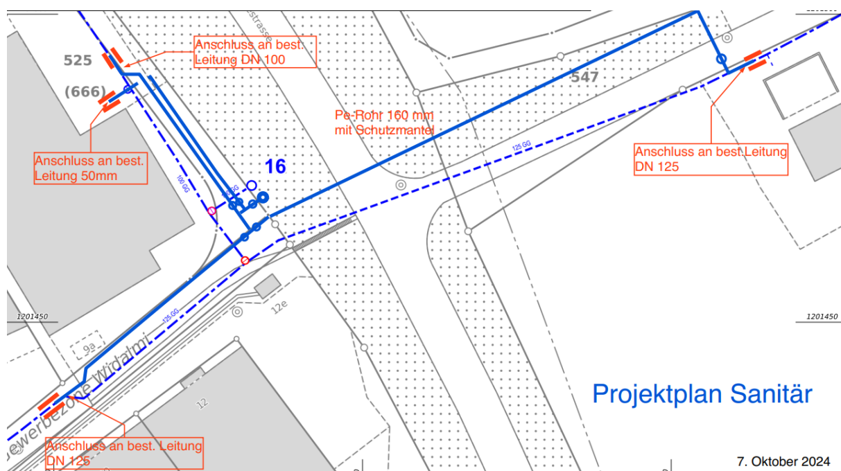
Bild: Projektplan Sanitär
