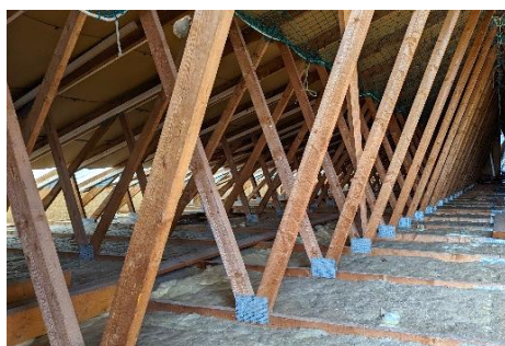
Dachkonstruktion und Modellverstärkung Turnhalle
