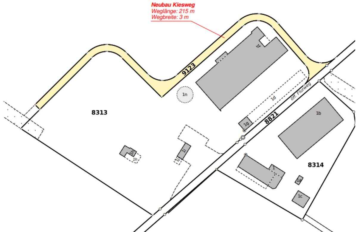
Situationsplan GeoPlanIng 2022 - Neuer Flurweg Kerzersmoos Parzelle 9123
